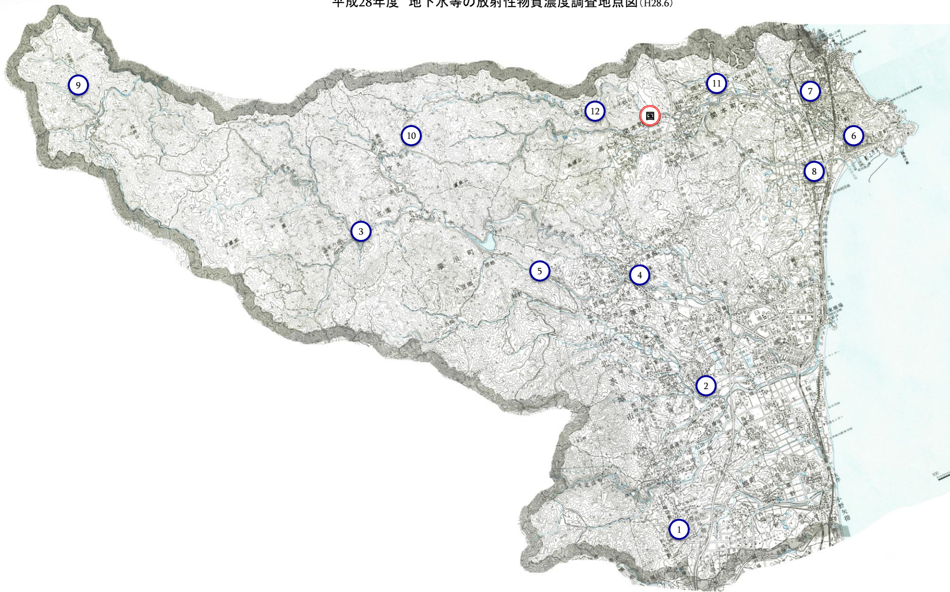
平成28年度 地下水等の放射性物質濃度調査地点図 (H28.6)
